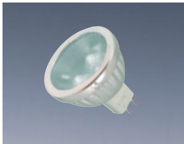
SL-206 MR-16 AC/DC 12V 消耗功率:5.0W / LED 4.2W Color:W / WW / R / G / B / Y 角度:156° 流明:225lm or 350lm (不定期提升)
