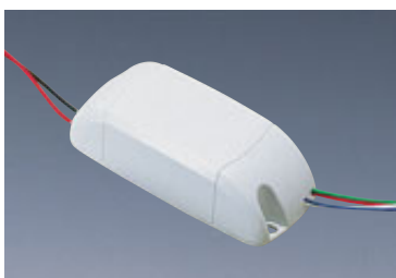
SC-1051變色訊號放大器 輸入:DC:12V / 輸出:30W 輸入:DC:24V / 輸出:60W 詳細規格請參考說明書
